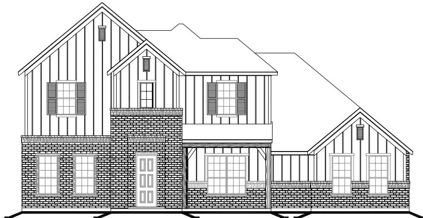
ELEVATION "C"
